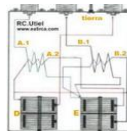
Acoplador Fig.52
